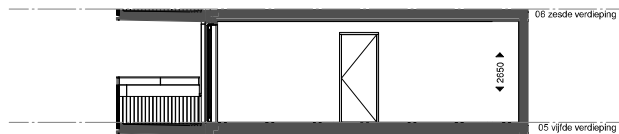
BNR 62 doorsnede
