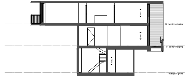
BNR 05 doorsnede
